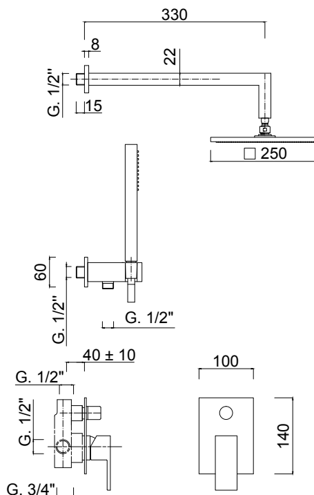
Soffione quadrato 250x250 mm Square showerhead 250x250 mm
