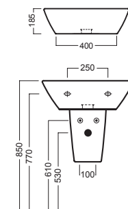
semicolonna_siphon cover
