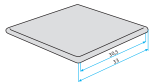
gradone toro angolare 33x33. 13"x13" ± 35 mm.
