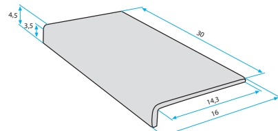
Elemento "L" 16x30x4,5. 6¼"x12"x1¼" ± 8,7 mm. solo su superficie matt for matt finish only
