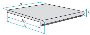
gradone toro vuoto bordo 30x33. 12"x13" ± 14 mm.
