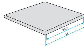
gradone toro vuoto angolare 33x33. 13"x13" ± 14 mm.
