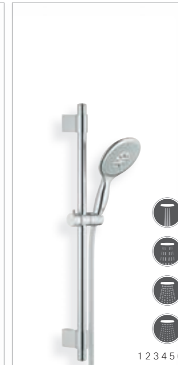
27 735 000 Set asta doccia completo asta 600 mm manopola doccia Ø 130 mm 27 736 000 con GROHE EcoJoy® a 9,5 l/min
