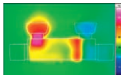
Immagine termica senza GROHE CoolTouch®
