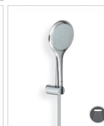
27 526 000 Set doccia completo manopola Ø 100 mm supporto a muro fisso 27 380 000 con GROHE EcoJoy® da 9,5 l/min.
