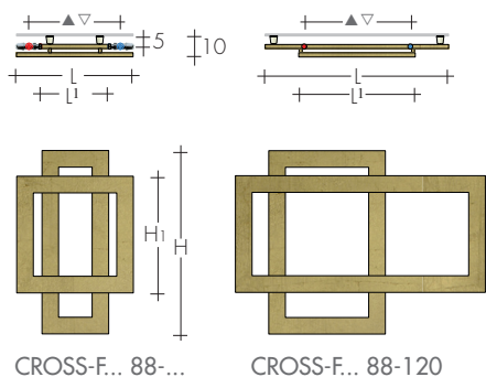
CROSS-F... 88-...
