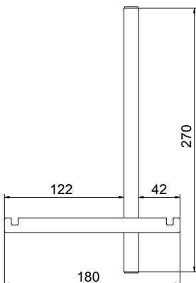
APPENDIABITI HOOK L. 180 x H. 270 mm
