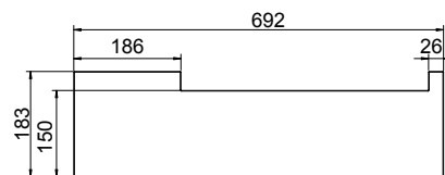
MENSOLA LEGNO WOOD SHELF L. 692 mm
